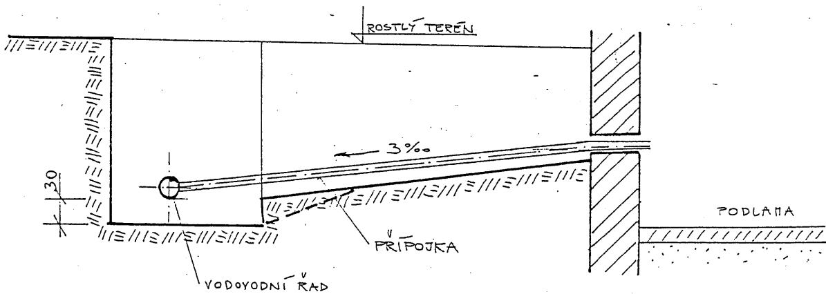
PODÉLNÝ ŘEZ
