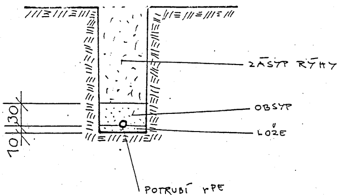
PŘÍČNÝ ŘEZ
